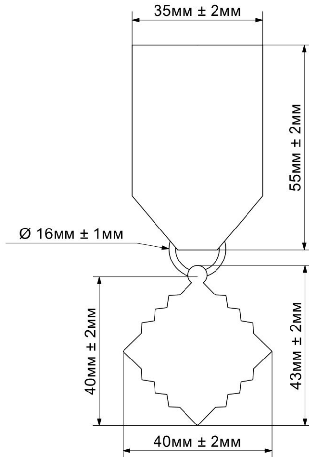
Рисунок Д1.2 – Лінійні розміри предмета
