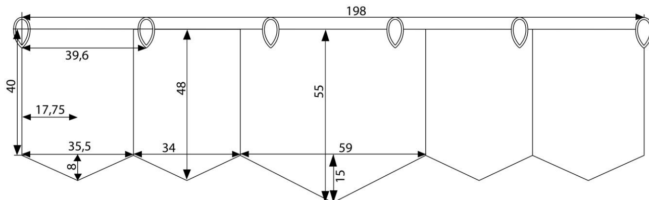
Рисунок Д1.4 – Розміри виробу 3 (Р-2)
