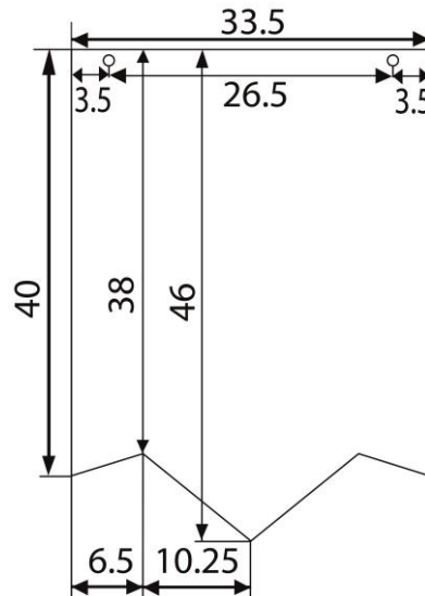
Рисунок Д1.1 – Розміри виробу 1
