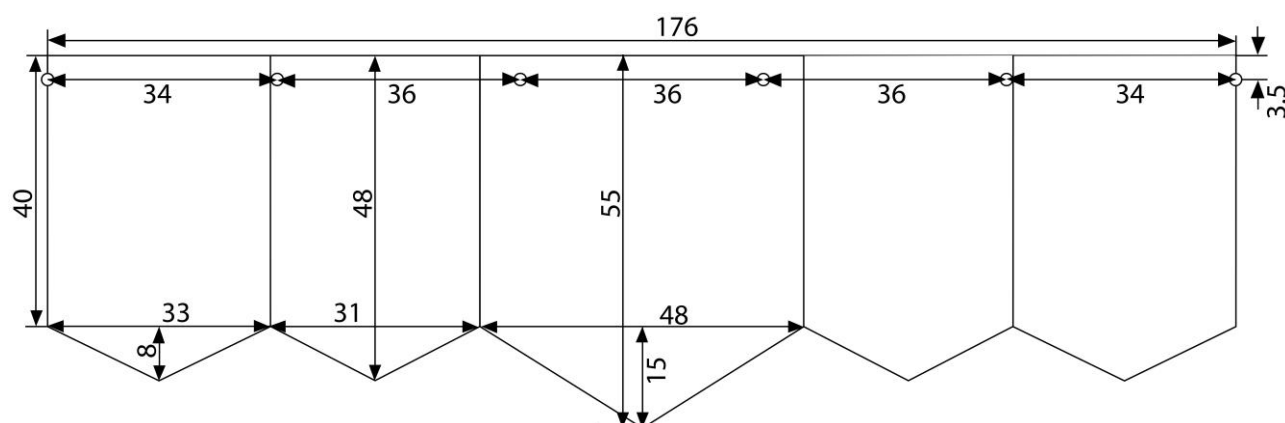
Рисунок Д1.6 – Розміри виробу 3 (Р-4)
