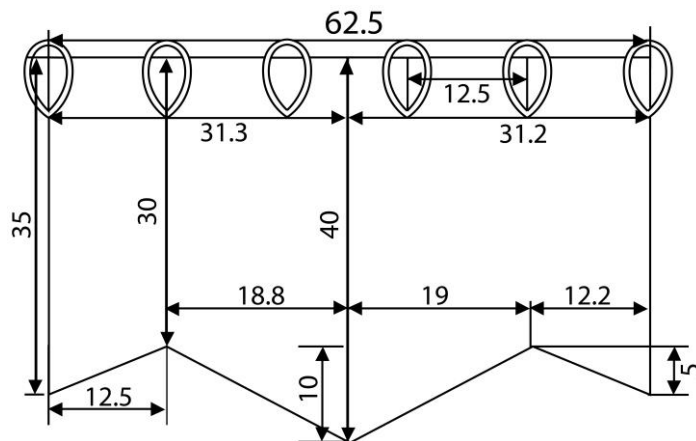
Рисунок Д1.2 – Розміри виробу 2
