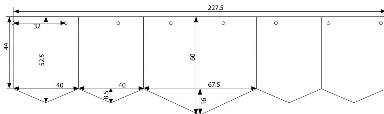
Рисунок Д1.5 – Розміри виробу 3 (Р-3)
