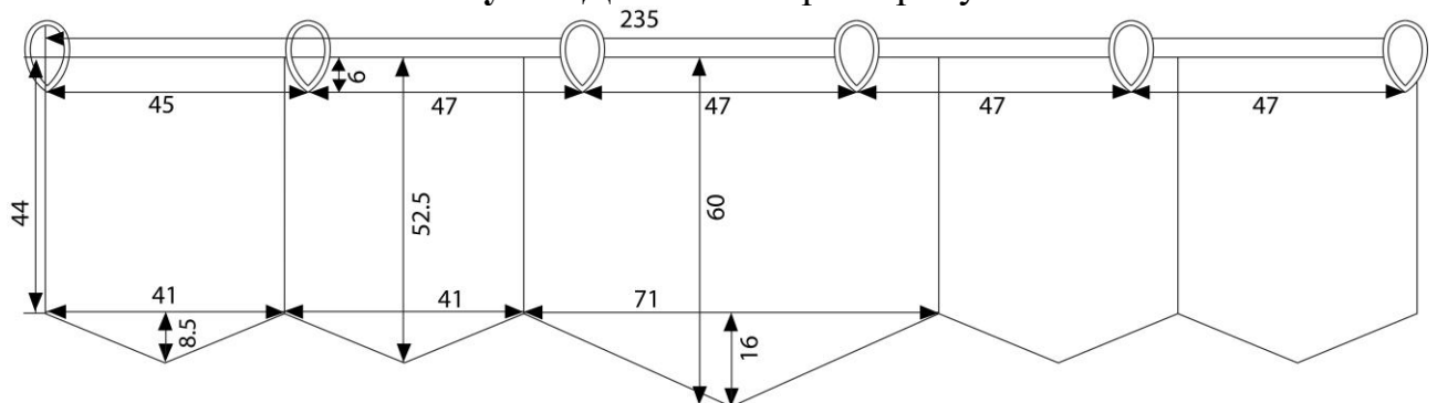
Рисунок Д1.3 – Розміри виробу 3 (Р-1)
