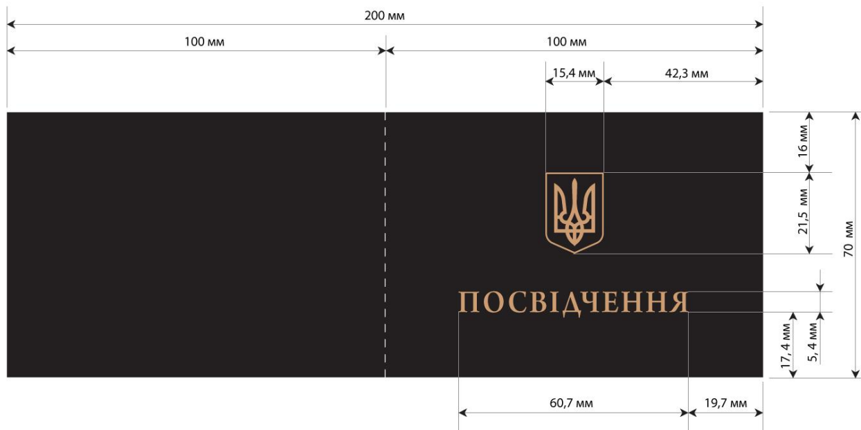
Рисунок Д2.1 – Лінійні розміри обкладинки предмета
