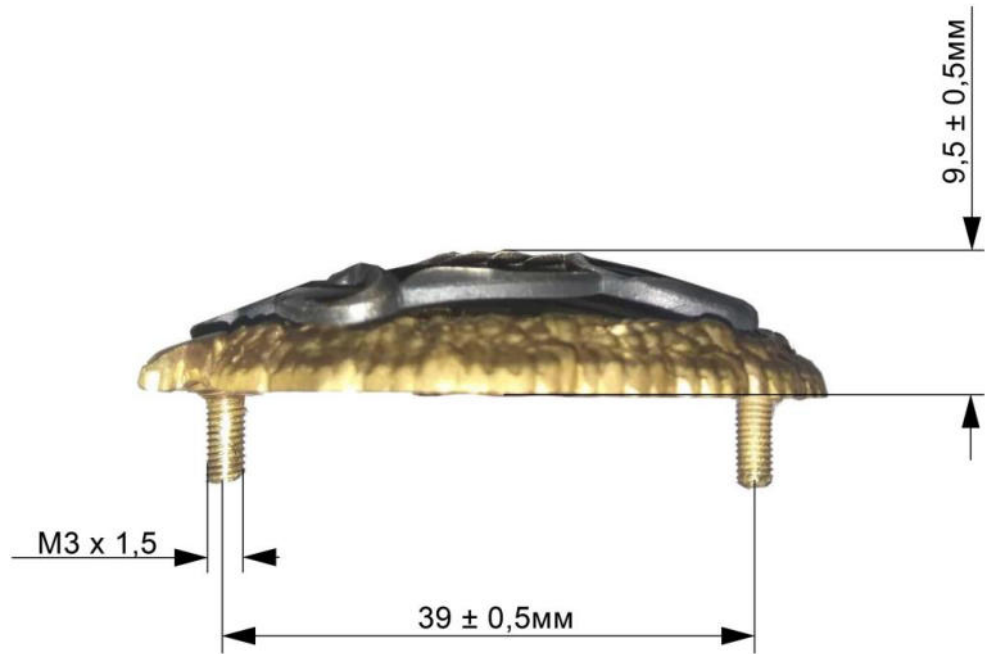
Рисунок Д3.1 – Розміщення кріплень знаку
