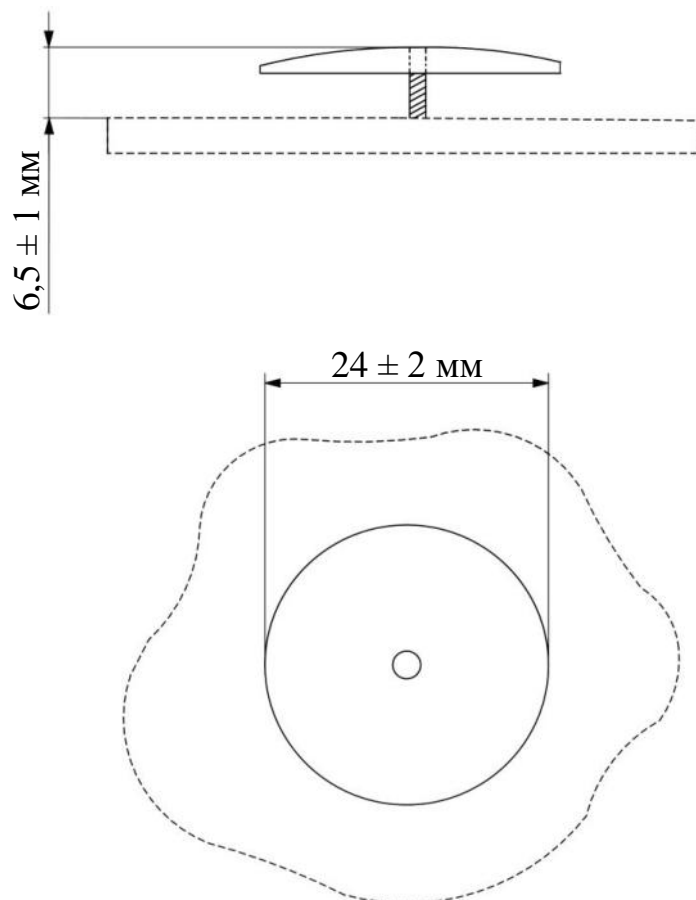
Рисунок Д3.1 – Розміри гвинта із закруткою
