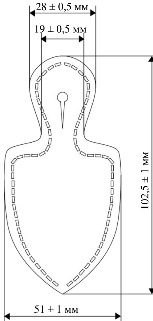
Рисунок Д1.1 – Розміри підкладки
