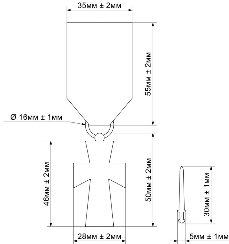
Рисунок Д1.3 – Лінійні розміри предмета
