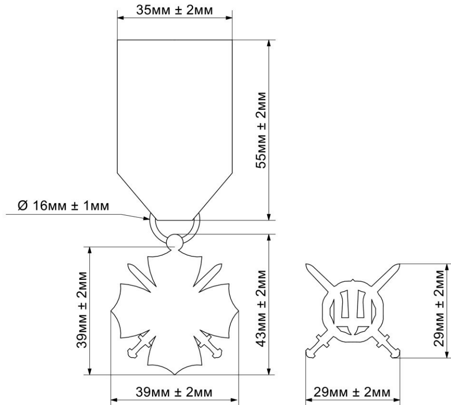
Рисунок Д1.3 – Лінійні розміри предмета
