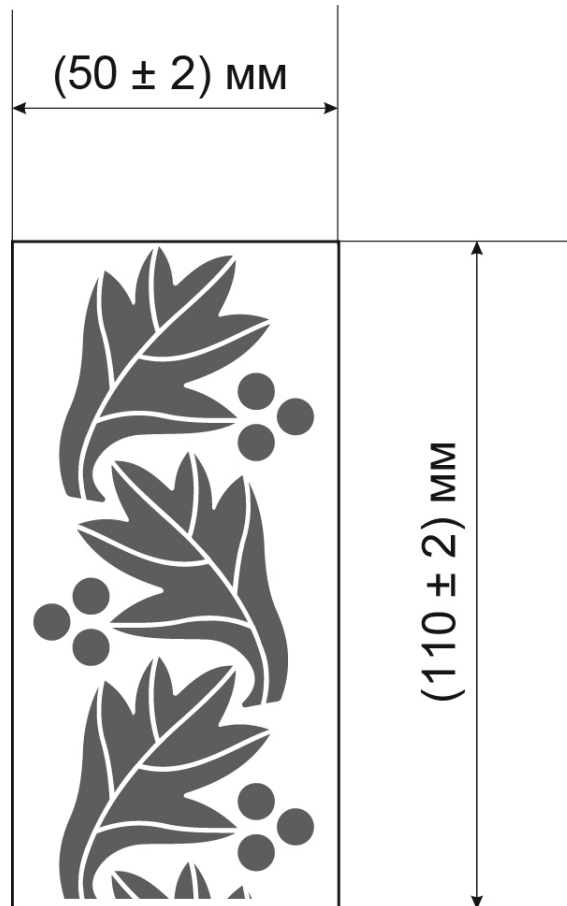
Рисунок Д1.1 – Розміри орнаменту
